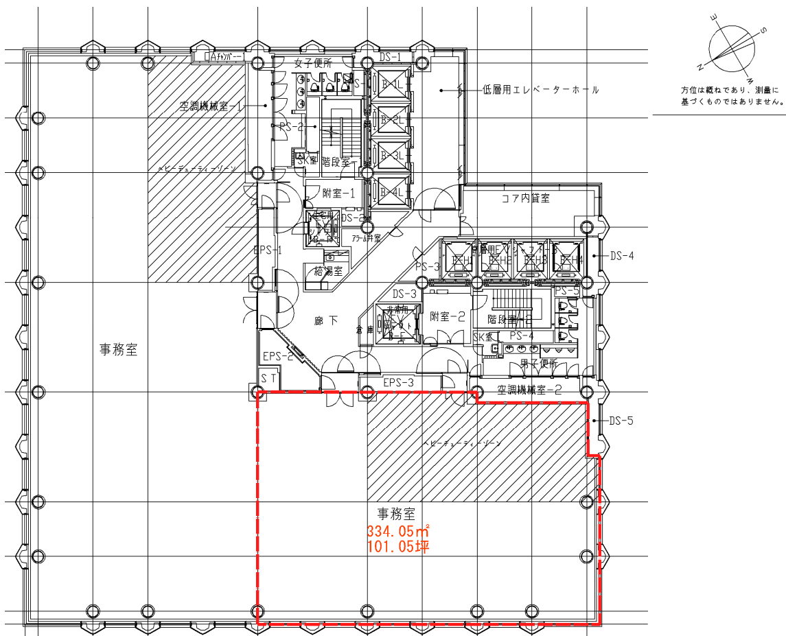
◆7階平面図
